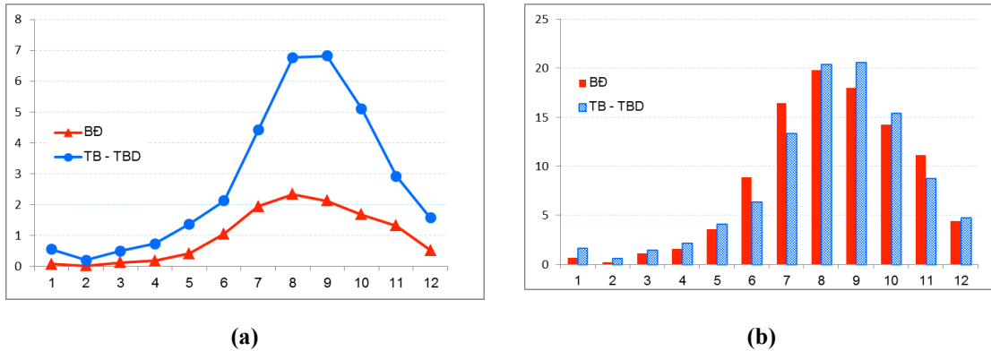
Hình 4. Số lượng XTNĐ trung bình tháng (hình a) và tỷ lệ % XTNĐ xảy ra ở các tháng trong năm (hình b) trên khu vực TBTBD và BD (thống kê số liệu RSMC, 1978-2015).
