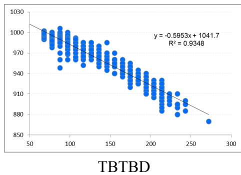
Hình 6. Mối quan hệ giữa P_{\min} (trục tung) và V_{\max} (trục hoành) của các XTNĐ trên khu vực TBTBD (hình trái) và BĐ (hình phải) (theo số liệu RSMC, 1978-2015).
