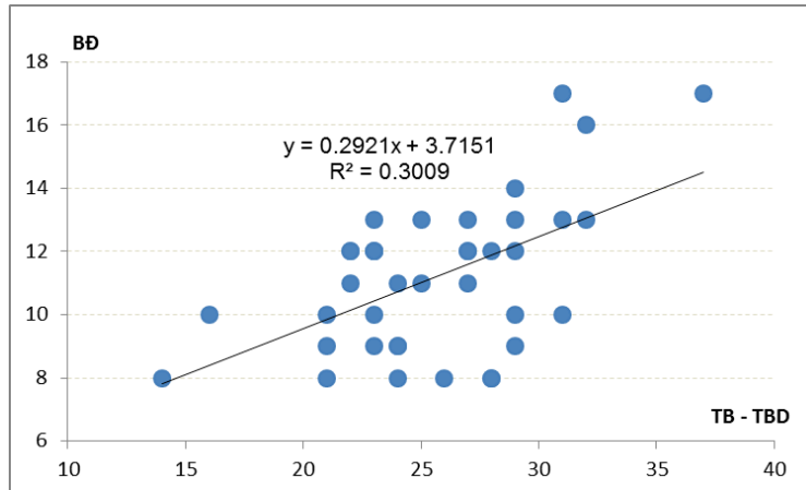
Hình 3. Mối quan hệ giữa số lượng XTNĐ giai đoạn 1978-2015 trên khu vực TBTBD và BD theo bộ số liệu RSMC.
